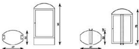
Dimensini del contenitore a terra e a palo
